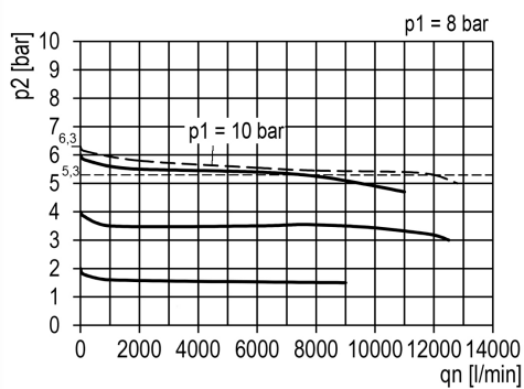
Durchflussdiagramm
